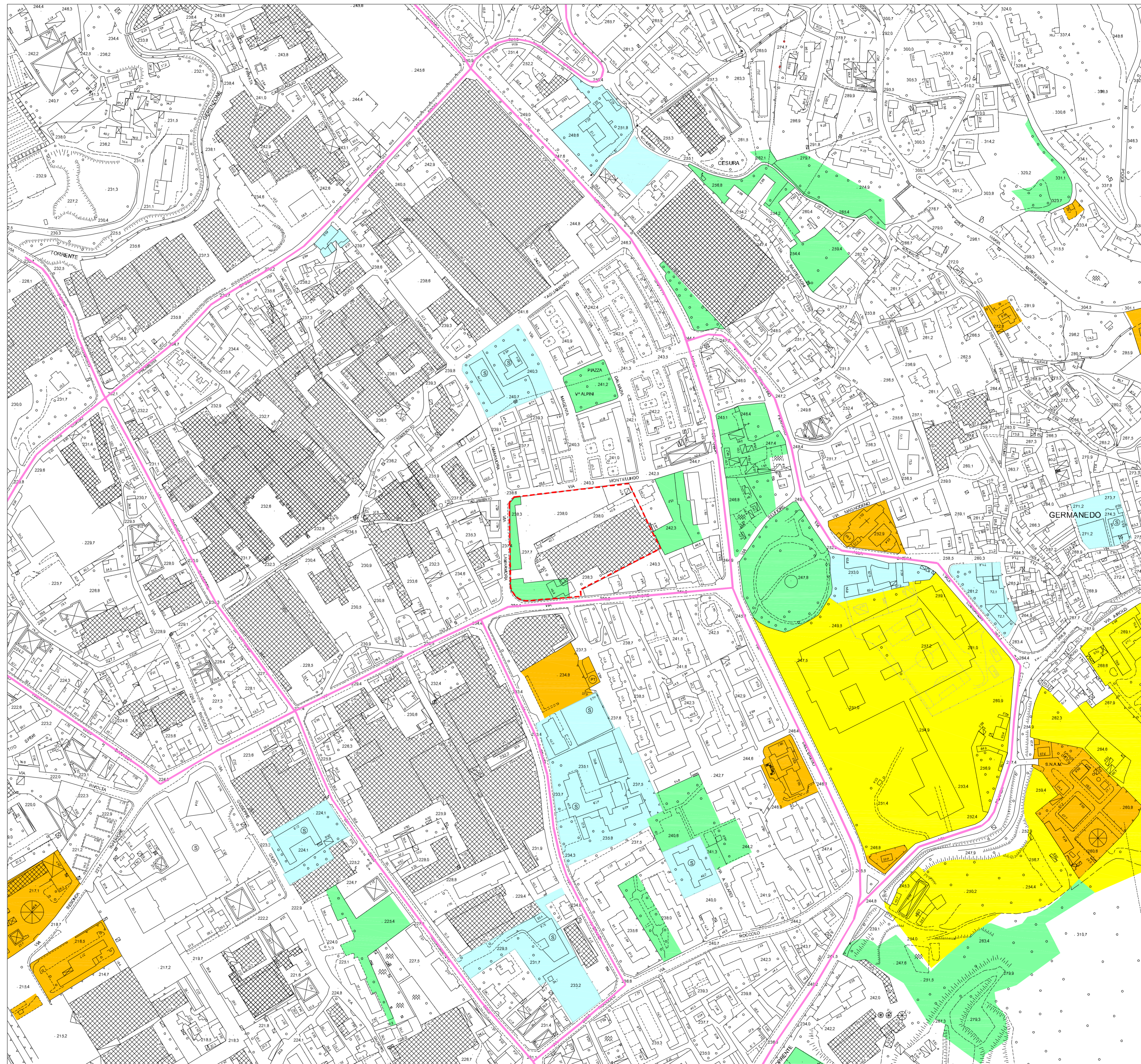
Stato attuale: inquadramento territoriale - scala 1:2000
